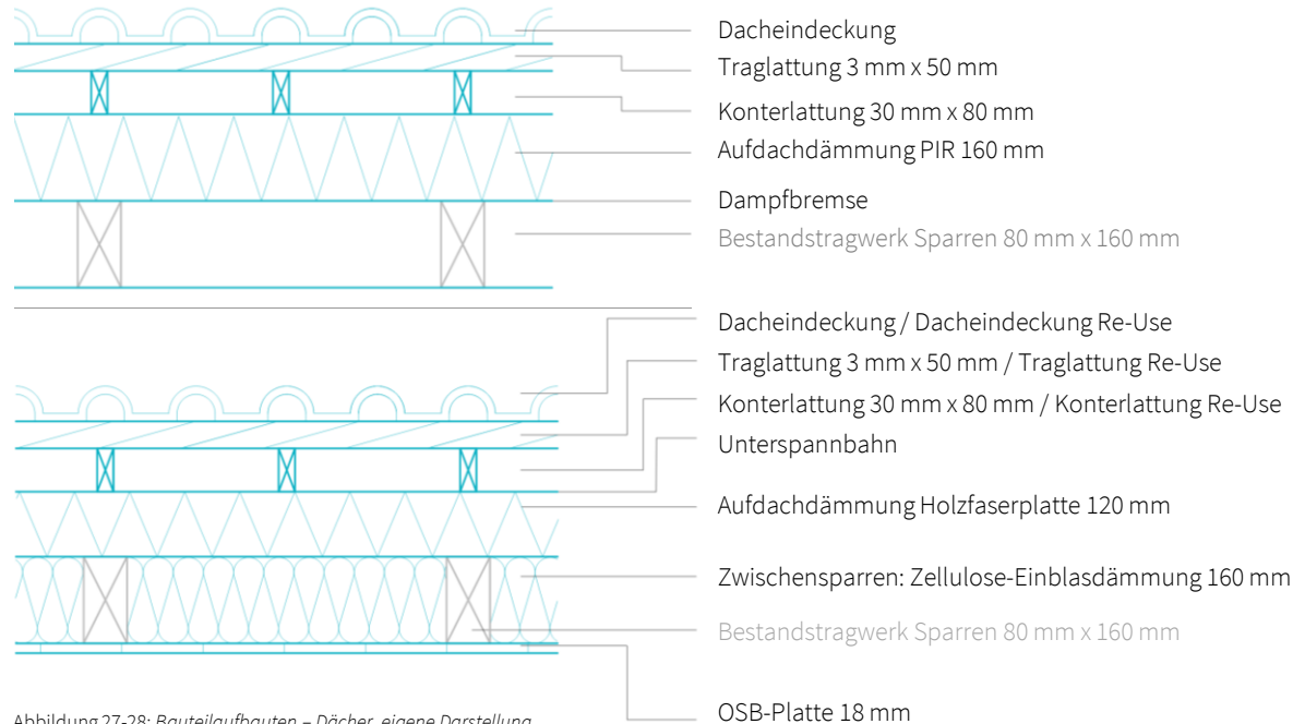
Abbildung 27-28: Bauteilaufbauten – Dächer, eigene Darstellung
