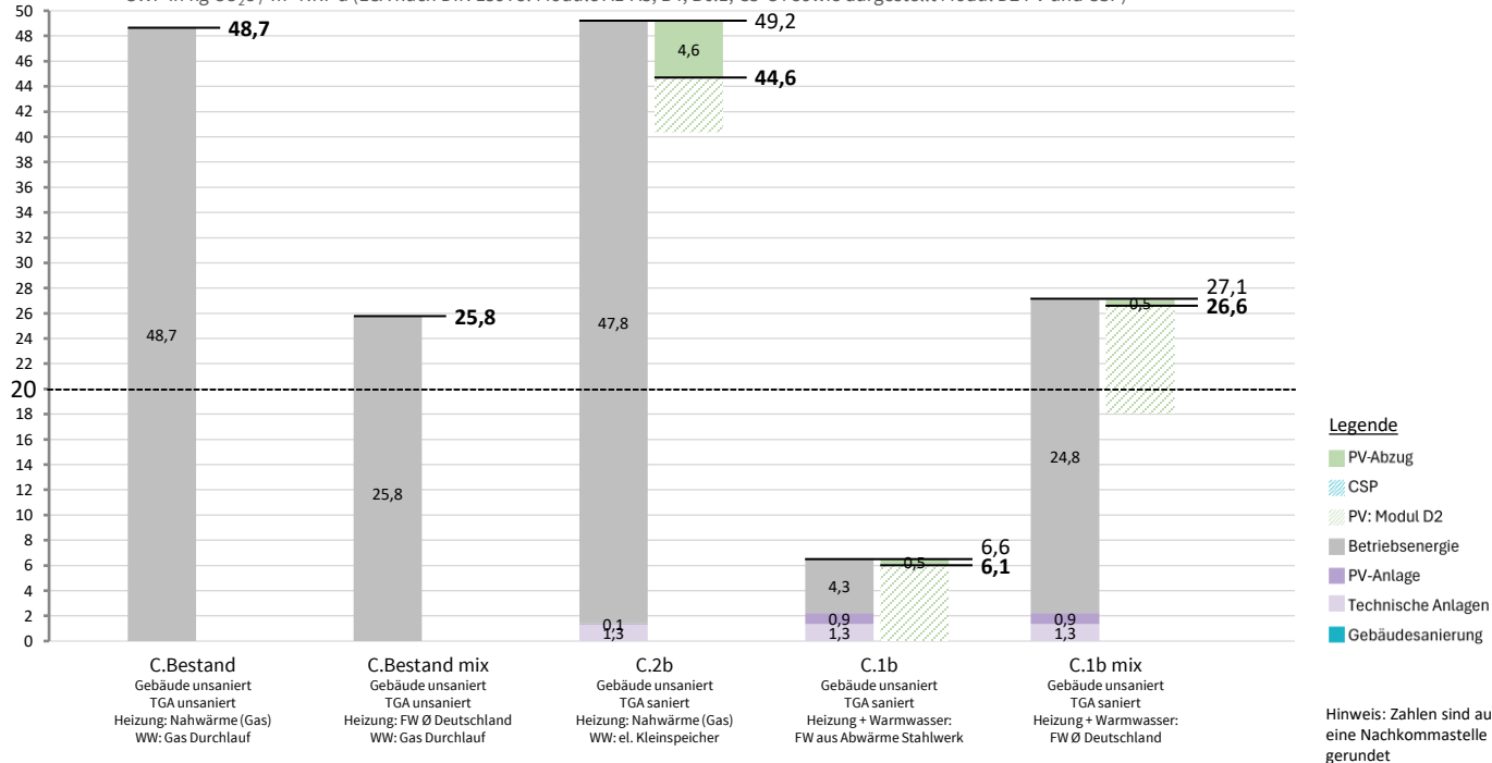
Abbildung 33: Ergebnisse LCA – Bestand mit Energiemix und Szenarien TGA Schäferkamp, eigene Darstellung
