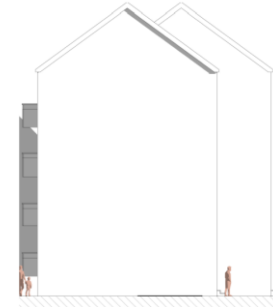
Ansicht Ost
