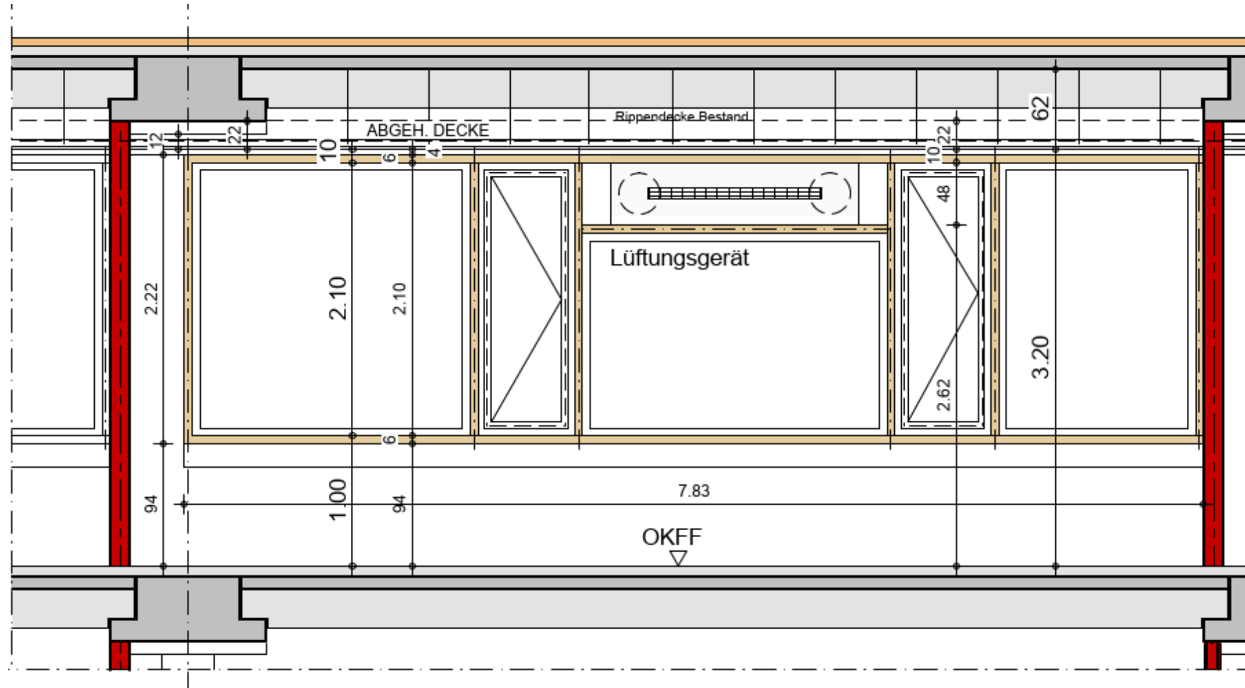
Innenansicht Klassenraum mit Lüftungsgerät
