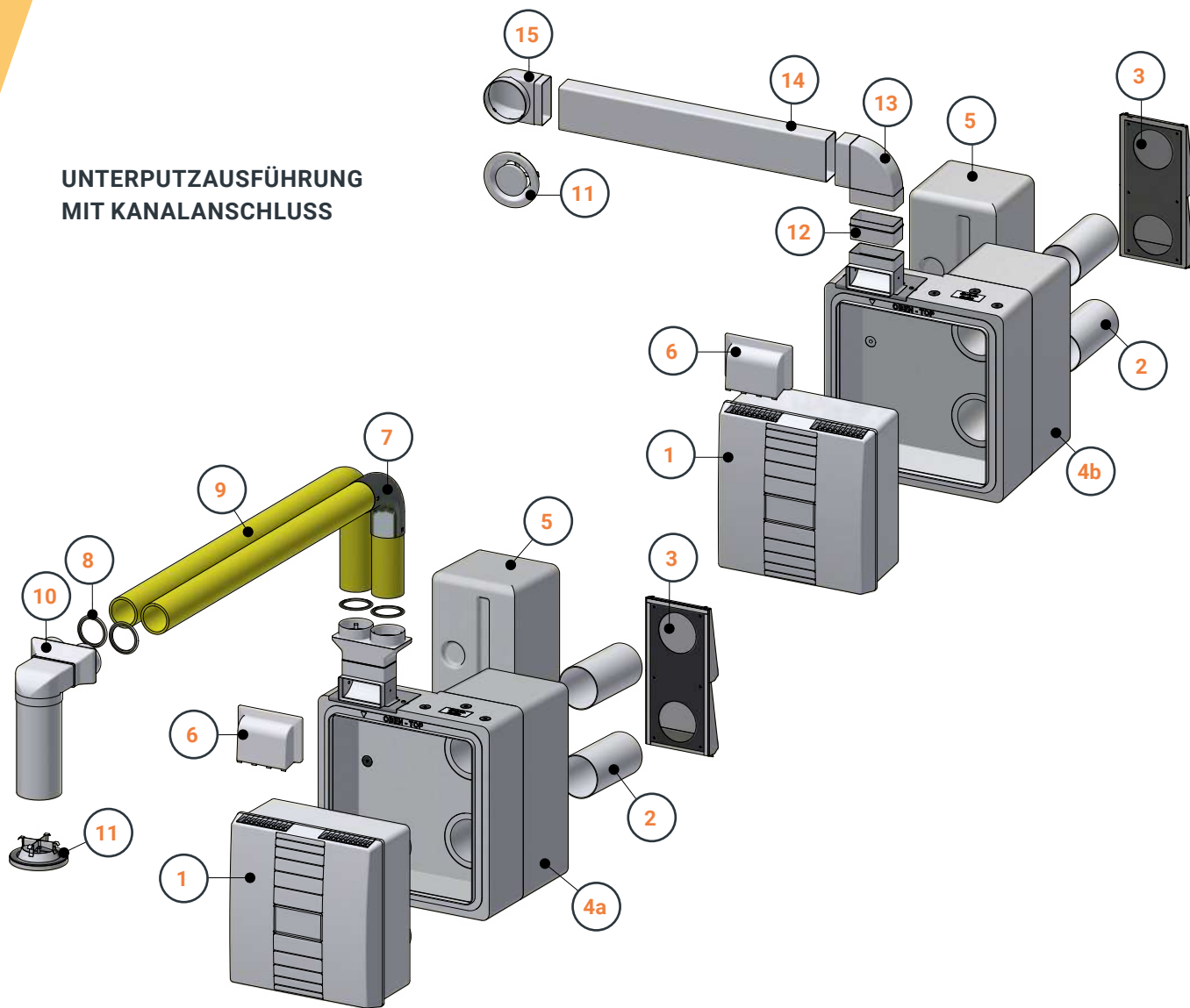
Bauteilliste
