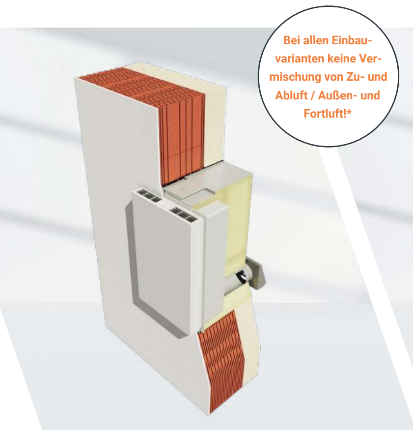
Wandintegrierter Einbau U² mit Kanalanschluss
