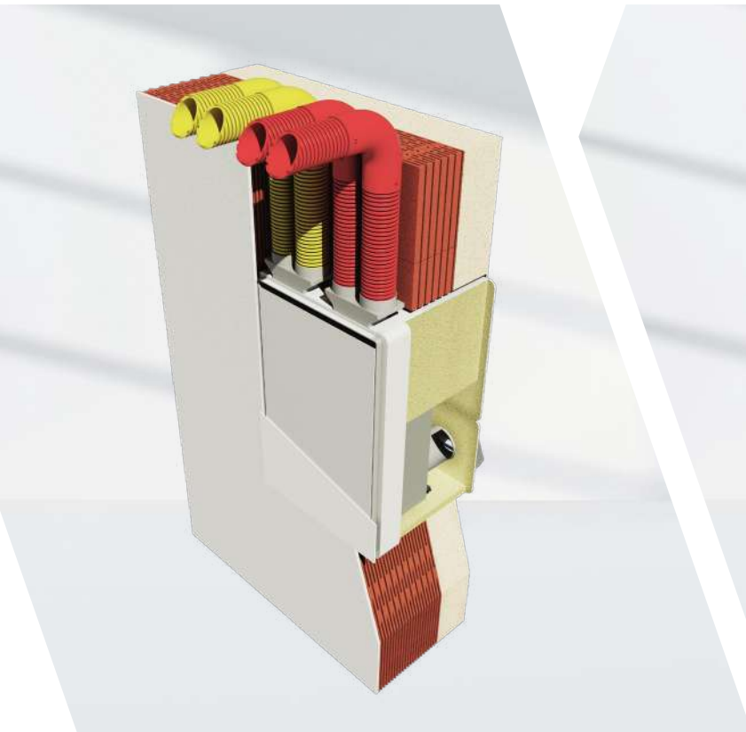
Wandintegrierter Einbau U² mit Kanalanschluss
