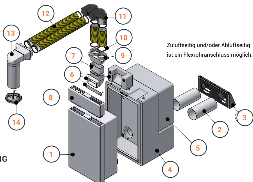
Bauteilliste
