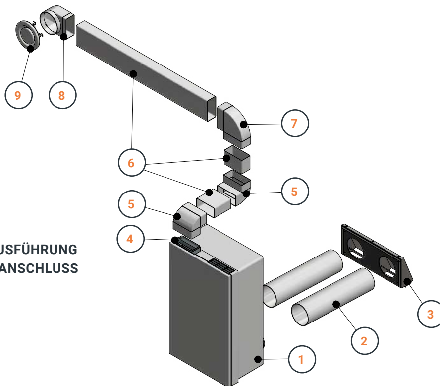
Bauteilliste
